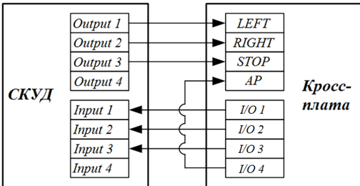
Рис. 10. Схема подключения пульта управления к контроллеру СКУД
